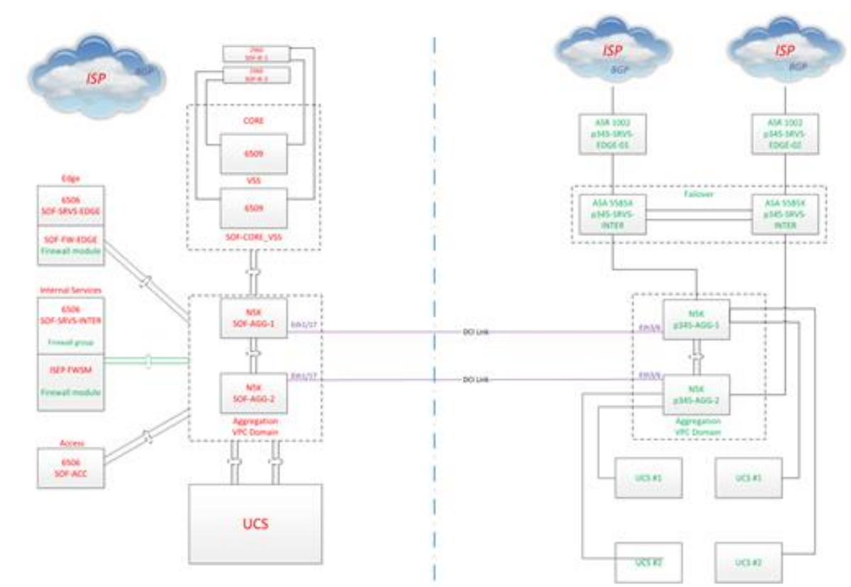
Принципна схема на свързаност на центровете за данни
